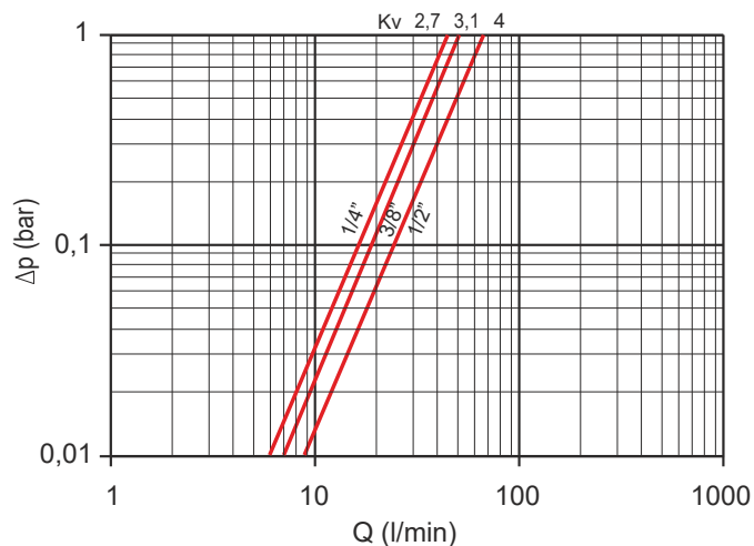
Диаграмма потерь давления
