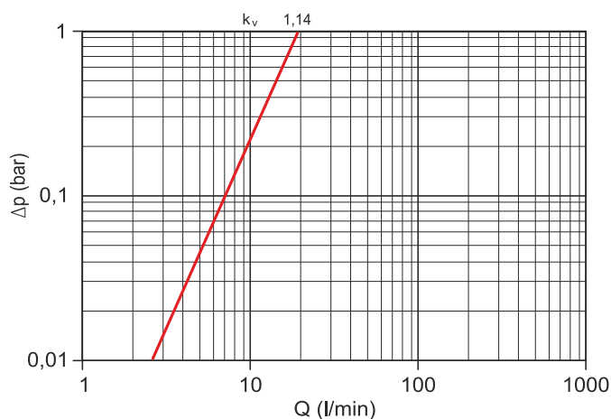
Диаграмма потерь давления
